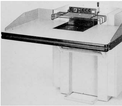
Sicherheitsabstand an einer Abfallzerkleinerungsmaschine durch großen Zuführtisch
