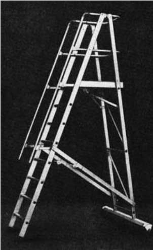
Podestleiter mit Handlauf – aufgestellt –
